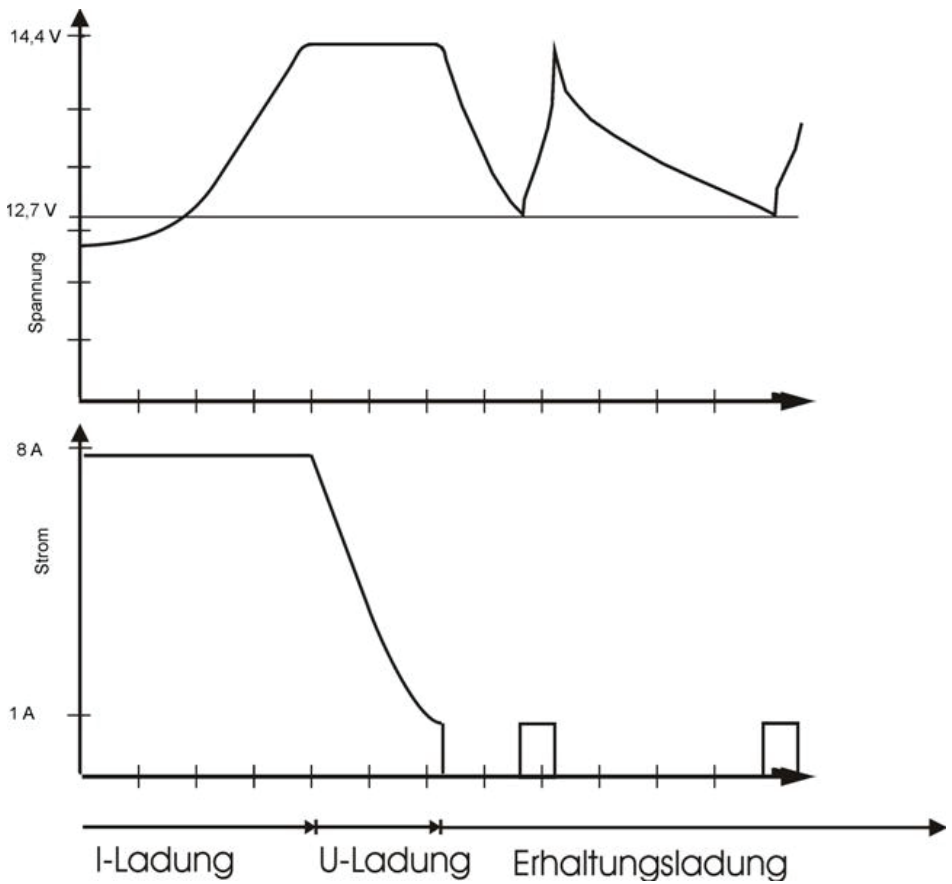
Typischer Ladespannungsverlauf (teilentladene, geschlossene 12V Bleibatterie)
